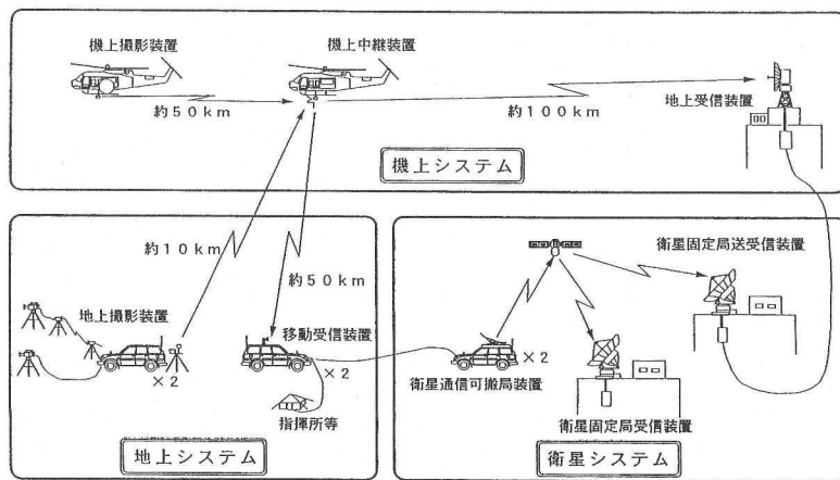
ヘリコプタ映像伝送装置構成図
