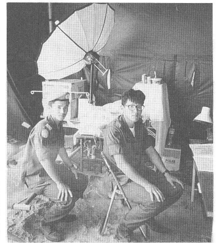
カンボディア タケオ駐屯地内の インマルサット衛星可搬型地球局
