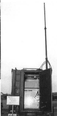
移動加入基地局装置
