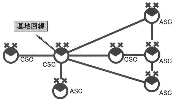
野外交換機 (SB-22)
